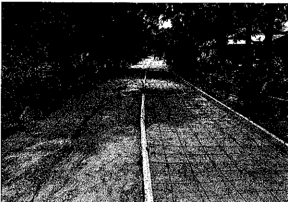
๒๗.โครงการก่อสร้างถนนคอนกรีตเสริมเหล็กยกพื้นสูง สายชอยกลางใจ หมู่ที่ ๔ บ้านโคกกล้วย ตำบลโชคเหนือ อำเภอลำดวน จังหวัดสุรินทร์
